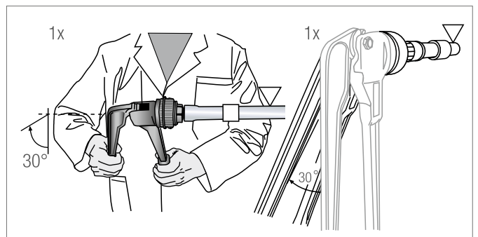
Abb. 10-7 Bei unveränderter Rohrlage Aufweitwerkzeug um 30° drehen und Rohr erneut aufweiten
