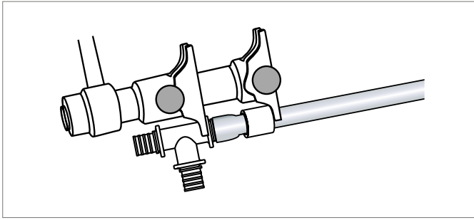
Abb. 10-10 Schiebehülsen-Verbindung in Verpresswerkzeug einsetzen
