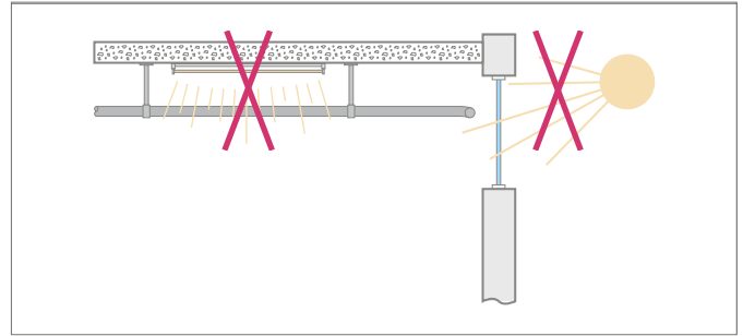
Abb. 17-7 Ungeschützte Verlegung im Bereich von UV-Strahlung nicht zulässig Beispiel Innenbereich
