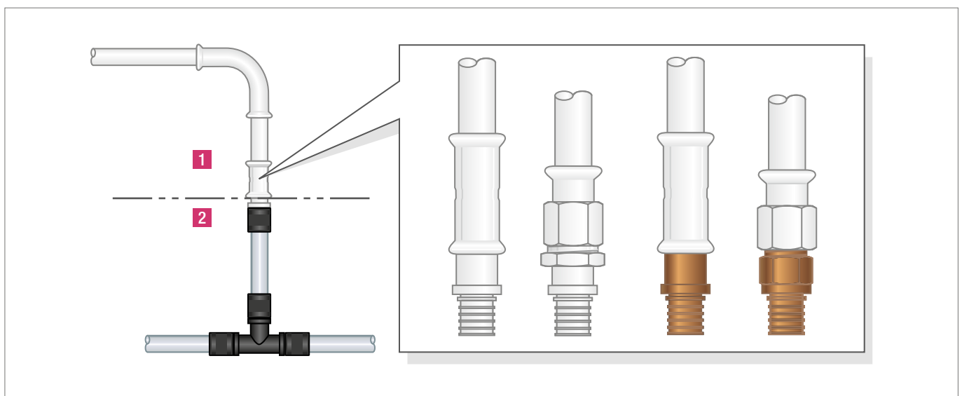
Abb. 6-21 Direkter Übergang von Edelstahlsystemen auf das System RAUTITAN bis zur Abmessung 32 oder bei Gewinden bis R1/Rp1 (Beispiel)
