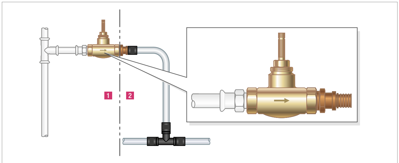
Abb. 6-20 Einbausituation Systemübergang an einem Unterputzventil (Beispiel)
