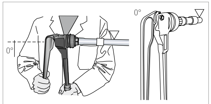
Abb. 10-6 Rohr einmal aufweiten
