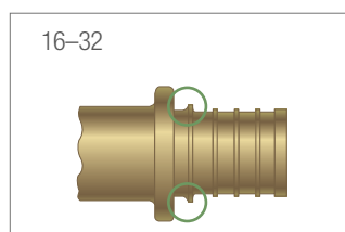
Abb. 19-3 Messing-Fitting, Voranschlag vollständig ausgeformt, Abmessung 16–32
