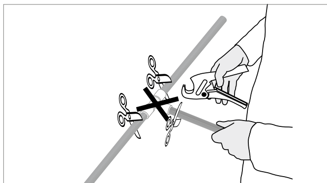
Abb. 11-1 Heraustrennen der Verbindung
