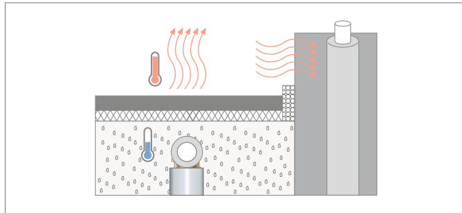
Abb. 17-11 Verlegung unter Heiasphaltestrichen
