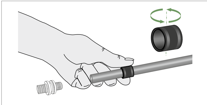
Abb. 10-2 Schiebehülse RAUTITAN PX über das Rohr schieben
