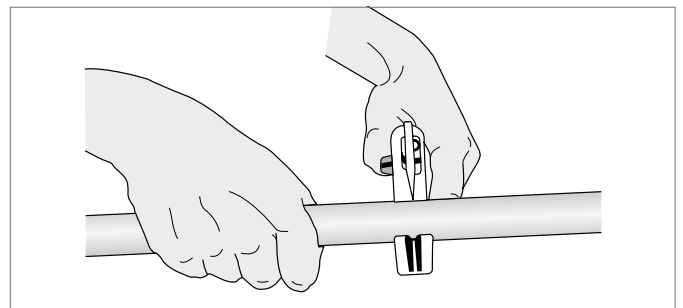
Abb. 10-1 Rohr rechtwinklig ablängen
