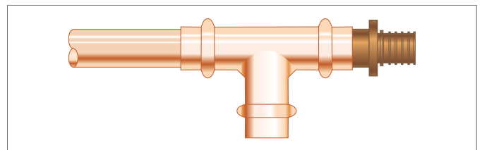
Abb. 6-16 Löt-Pressübergang RAUTITAN RX mit Kupferpresssystem
