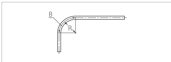
Abb. 12-2 Biegeradius und Bogenmaß
