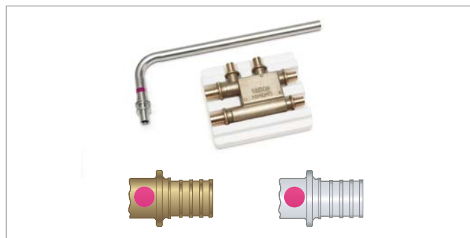
Abb. 6-6 Fittings ausschließlich für die Heizungsinstallation
