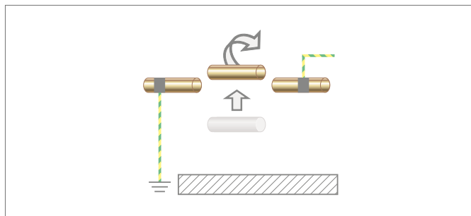
Abb. 17-12 Potenzialausgleich beim Austausch von Rohren
