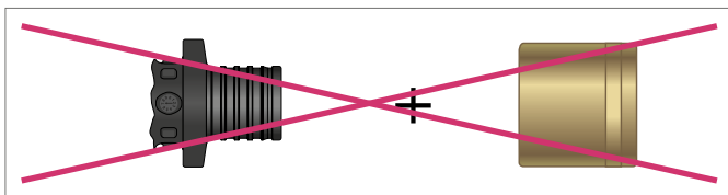
Abb. 10-4 Unzulässige Kombination RAUTITAN PX mit RAUTITAN Messingschiebehülsen
