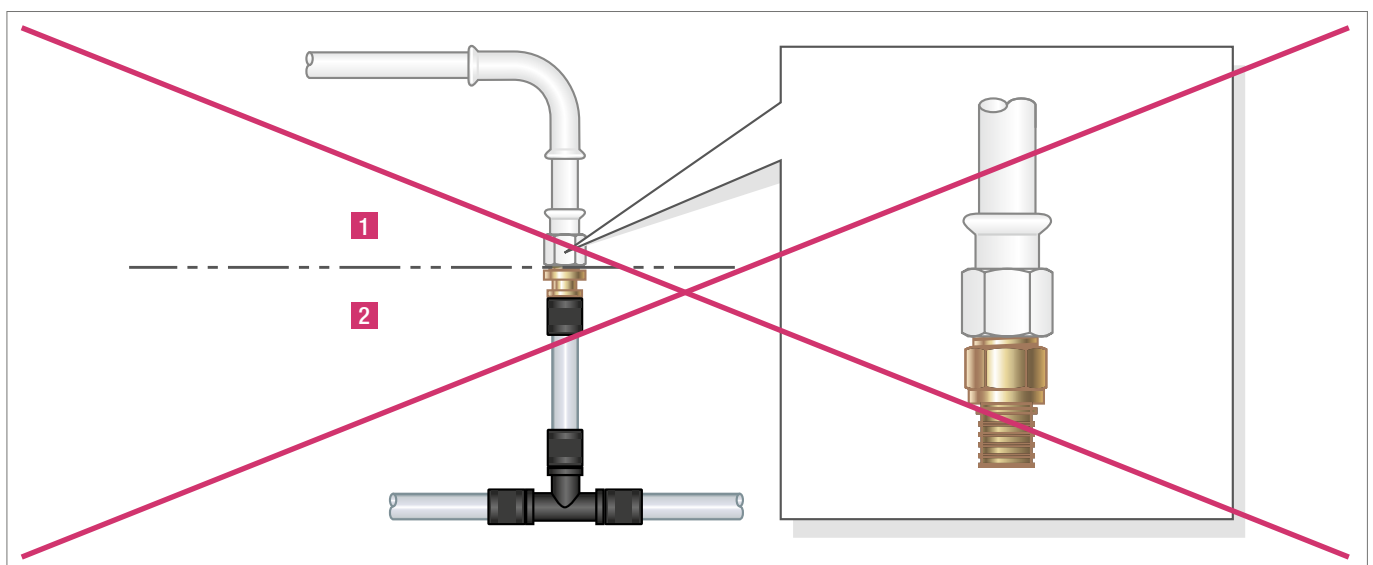
Abb. 6-22 Kein direkter Übergang von Edelstahlsystemen mit RAUTITAN MX
