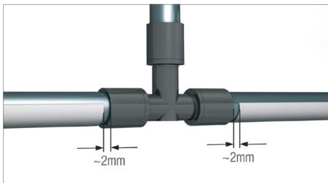
Abb. 13-5 Schiebehülsen RAUTITAN PX nicht überclippen
