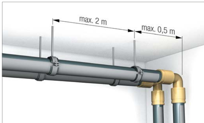
Abb. 13-3 Maximale Rohrschellenabstände
