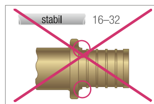
Abb. 19-2 Messing-Fitting, Voranschlag teilweise ausgeformt, Abmessung 16–32
