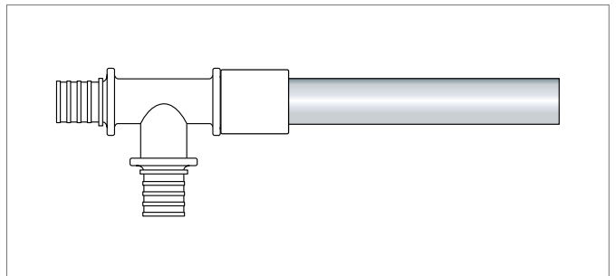
Abb. 10-12 Fertig verpresste Schiebehülsen-Verbindung
