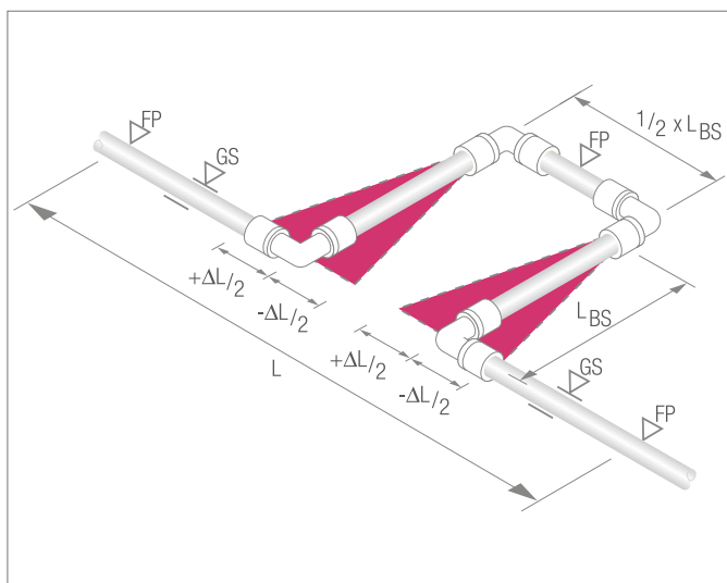
Abb. 16-2 U-Dehnungsbogen
