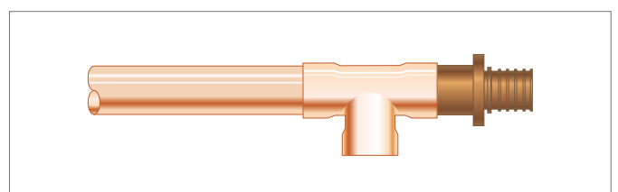
Abb. 6-17 Löt-Pressübergang RAUTITAN RX eingelötet in Kupferrohrsystem
