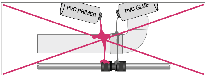
Abb. 6-27 RAUTITAN PX: Kontakt mit Kleber wie PVC-Kleber vermeiden
