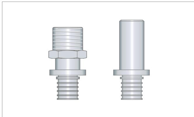
Abb. 6-19 Systemübergang mit Außengewinde RAUTITAN SX aus Edelstahl und System-Pressübergang RAUTITAN SX aus Edelstahl
