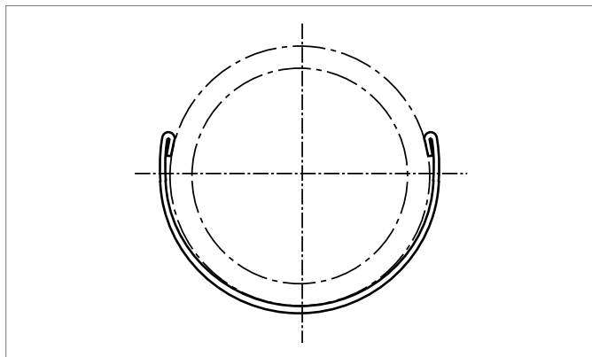
Abb. 13-1 Querschnitt Cliphalschale
