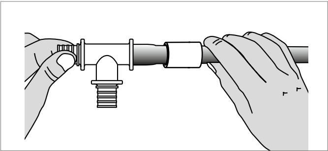
Abb. 10-8 Fitting in das aufgeweitete Rohr stecken
