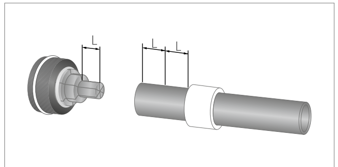
Abb. 10-5 Mindestabstand Rohrende – Schiebehülse
