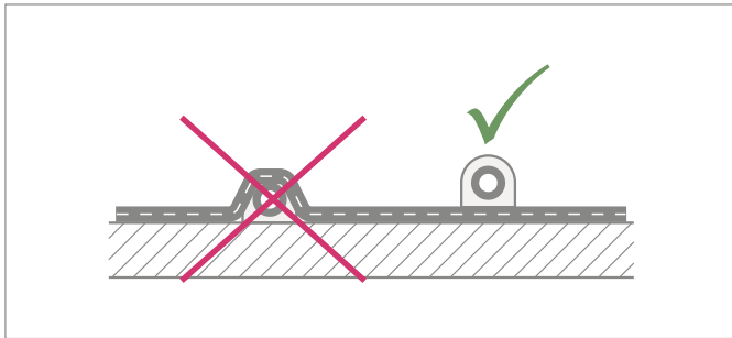
Abb. 17-9 Verlegung nur auf einer Bitumenbahn zulässig
