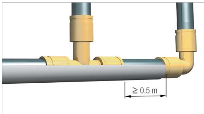
Abb. 13-4 Mindestüberlappung von 0,5 m
