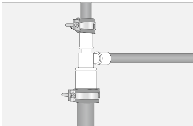
Abb. 14-1 Festpunkt ausgeführt mit Rohrschellen
