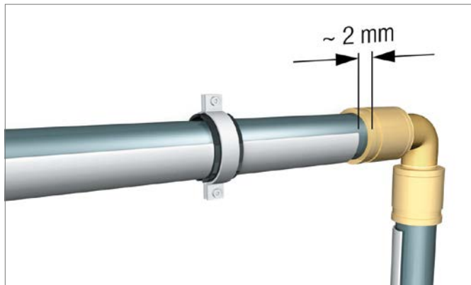
Abb. 13-2 Cliphalschale ca. 2 mm vor Schiebehülse enden lassen
