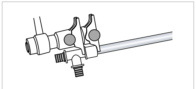
Abb. 10-11 Schiebehülse aufschieben
