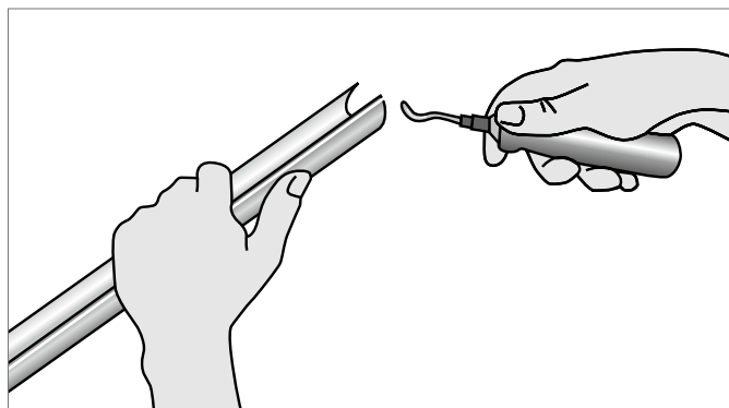
Abb. 13-7 Entgraten
