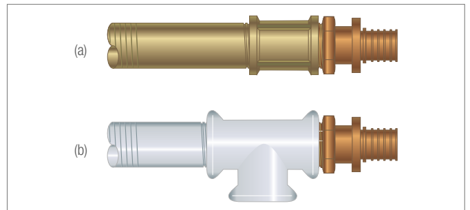
Abb. 6-15 Übergang mit Außengewinde RAUTITAN eingeschraubt in: (a) Messingfittings (b) Systeme mit verzinkten Rohren und Fittings
