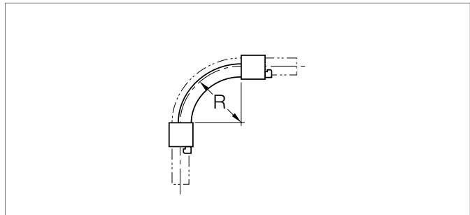
Abb. 12-6 Rohrführungsbogen Sanitär 90 Grad, für Abmessung 16–32 und Rohrführungsbogen Sanitär/Heizung 5 x d 90 Grad für Abmessung 32 R Biegeradius
