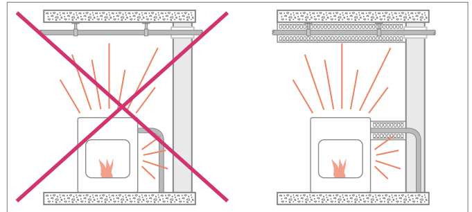
Abb. 17-3 Schutz vor thermischer Belastung
