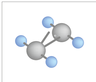
Abb. 5-2 Ethylen, aufgehende Doppelverbindung
