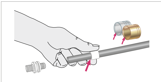
Abb. 10-3 Schiebehülse aus Messing über das Rohr schieben, innere Anfasung (Pfeil) zeigt zur Verbindung
