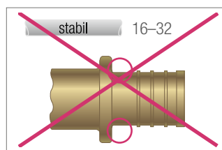
Abb. 19-1 Messing-Fitting, Voranschlag nicht ausgeformt, Abmessung 16–32
